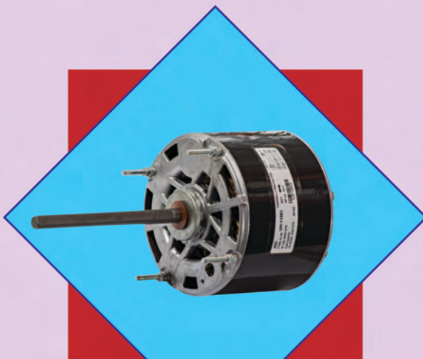
ARAH-UH-11061 A/C PICL OUT DOOR FAN MOTOR CARRIER LONG SHAFT 1/4HP 5 UF
