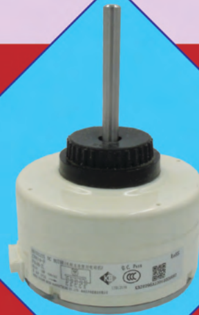
ARAH-ZWR50-F SPLIT A/C INDOOR FAN MOTOR 50W
